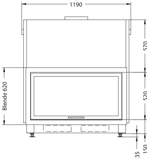
Vorderansicht M~1:20
