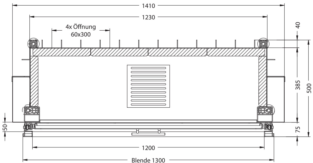
Horizontalschnitt M~1:10
