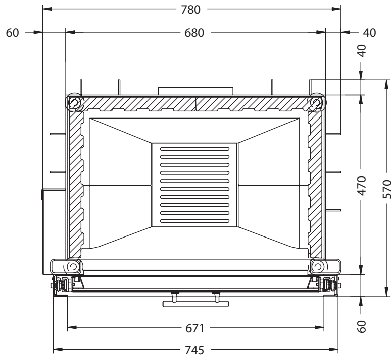
Horizontalschnitt M~1:10
